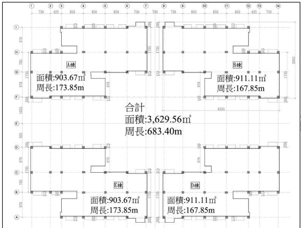
平面形狀係數 f_1 參數檢討圖
