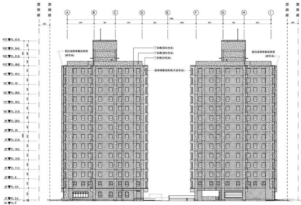
西向立面圖
