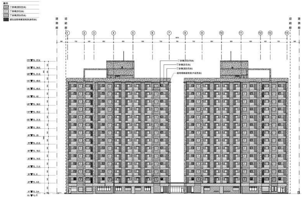
南向立面圖
