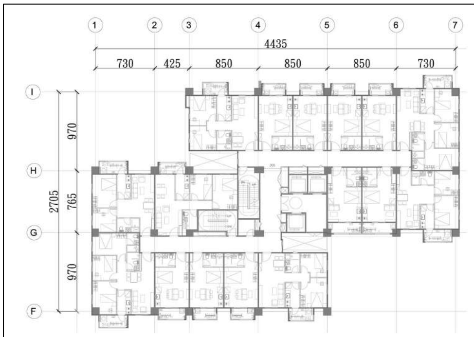
跨距比解析圖
