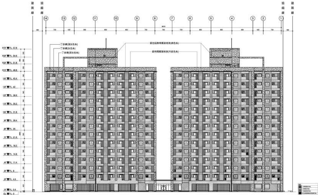
北向立面圖
